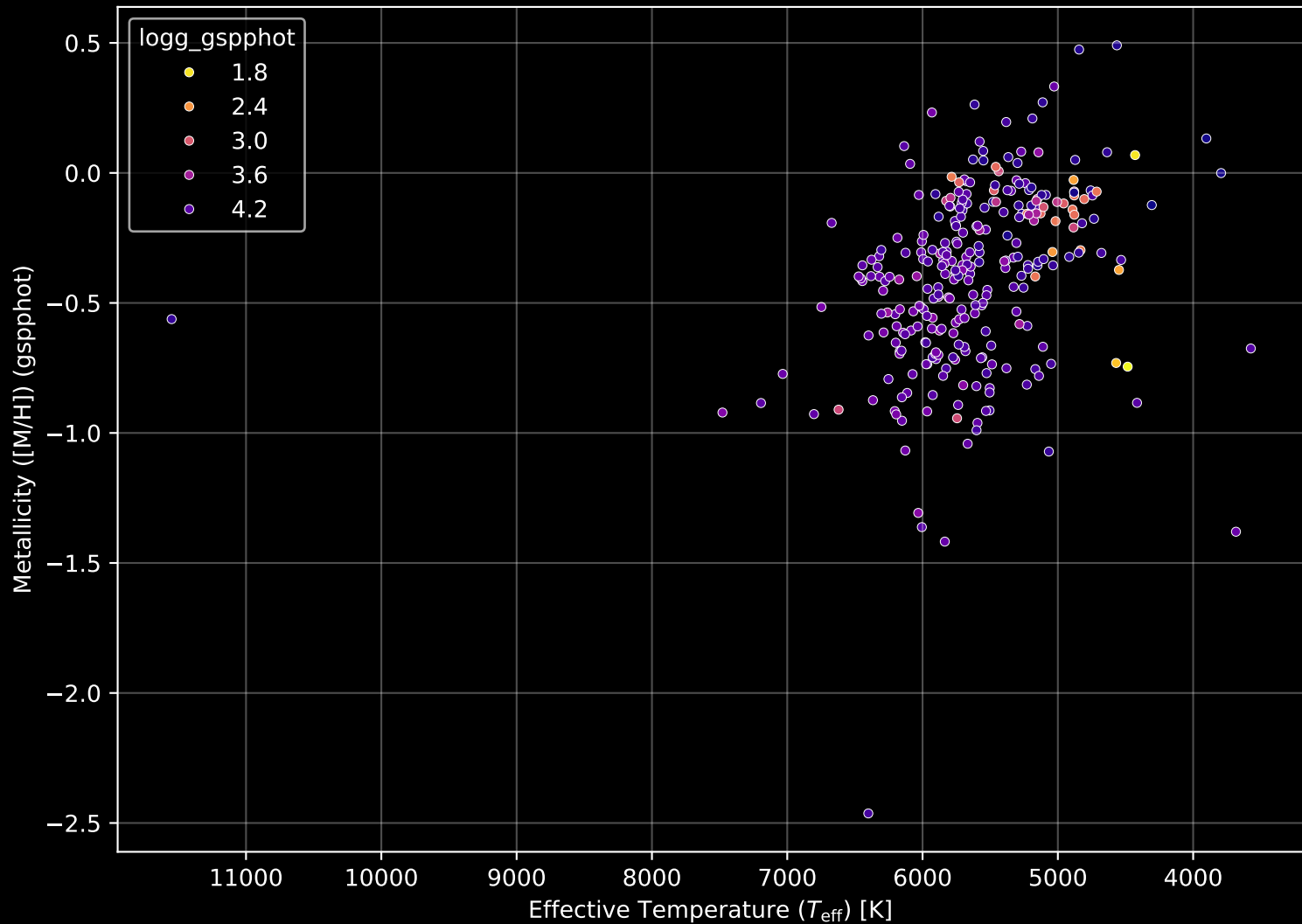
GALAH DR4 Field: [287] Stellar Population Parameters (n= 291)
