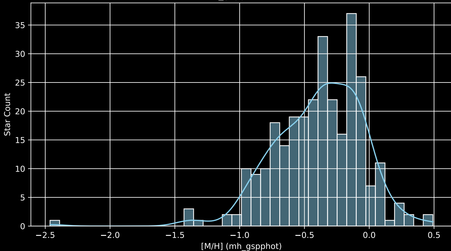
GALAH DR4 Field: [287] [M/H] (mh_gspphot) (n= 291)
