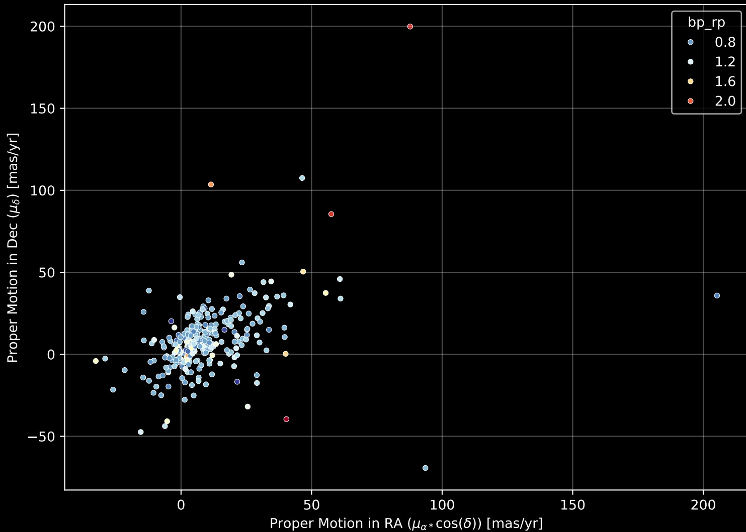
GALAH DR4 Field: [287] Proper Motion Diagram (n= 291)
