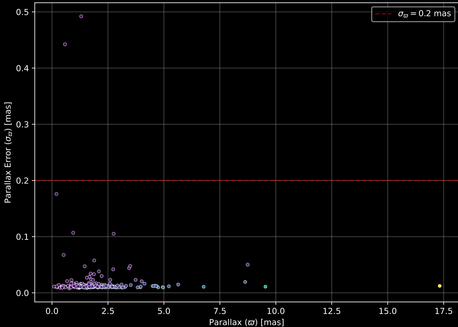
GALAH DR4 Field: [287] Parallax Quality (n= 291)
